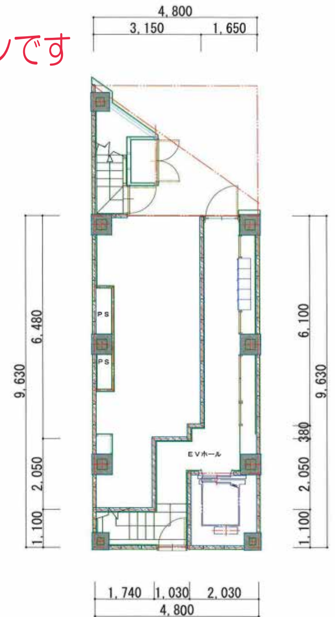
1階平面図
