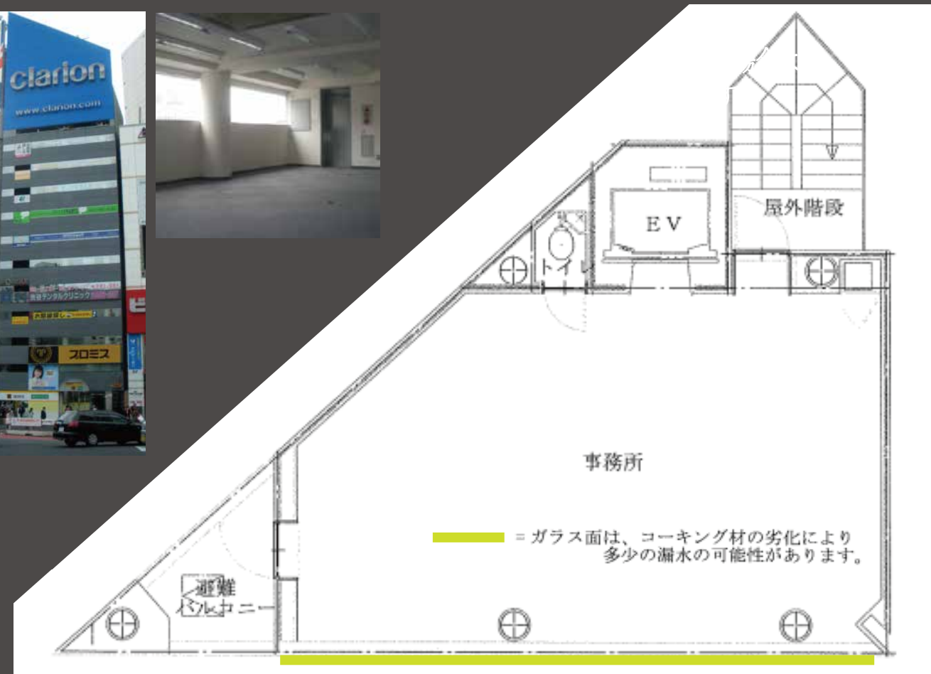
【6階 平面図】
