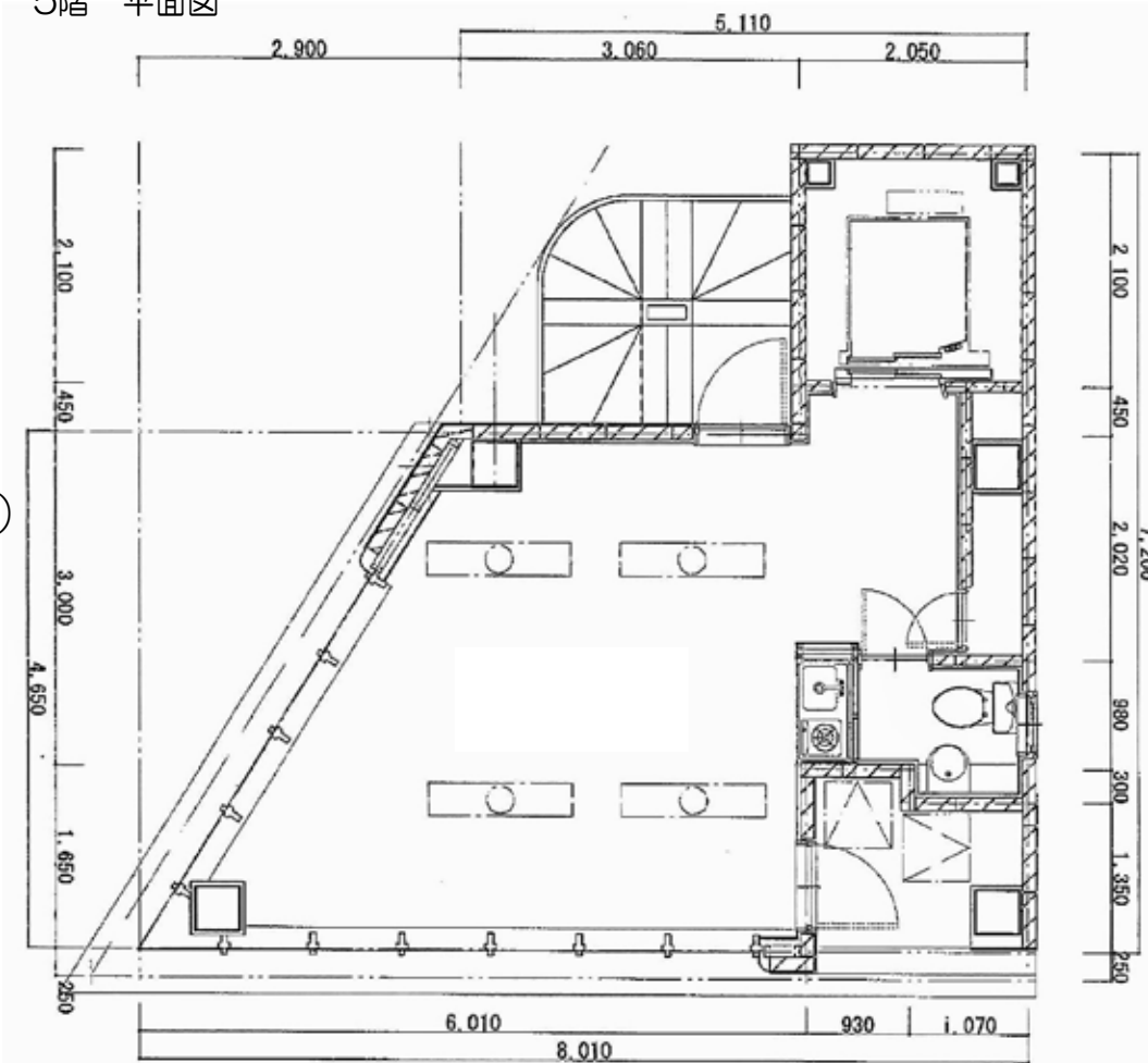
5階 平面図
