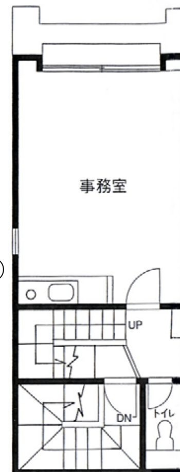
5階平面図
