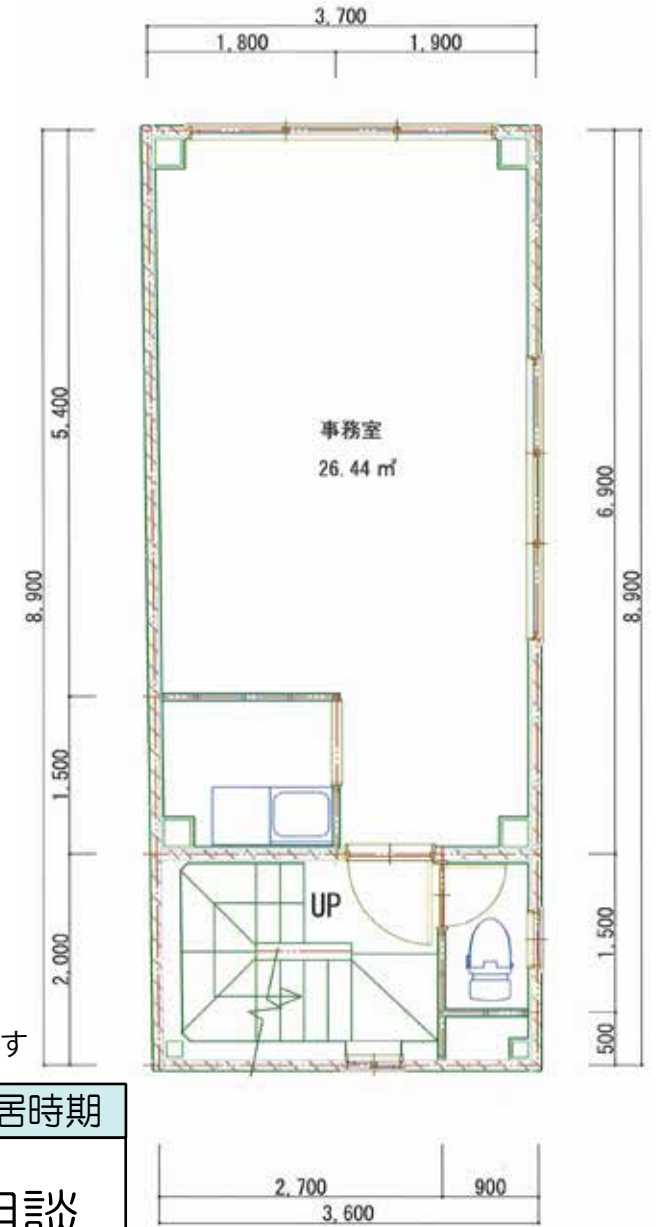
【2階 平面図】
